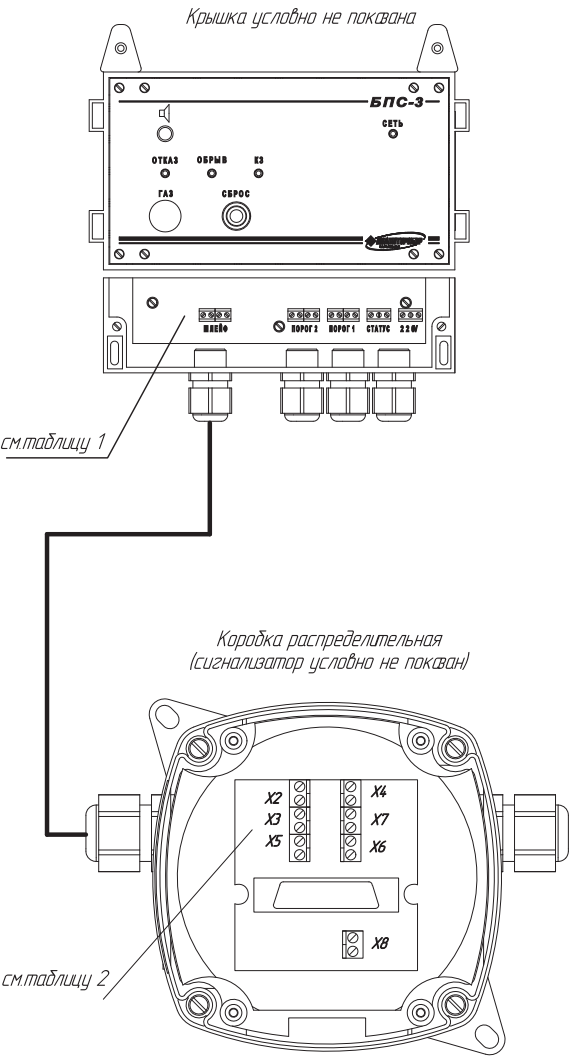
а) сигнализатор СТГ-3 с блоком БПС-3
