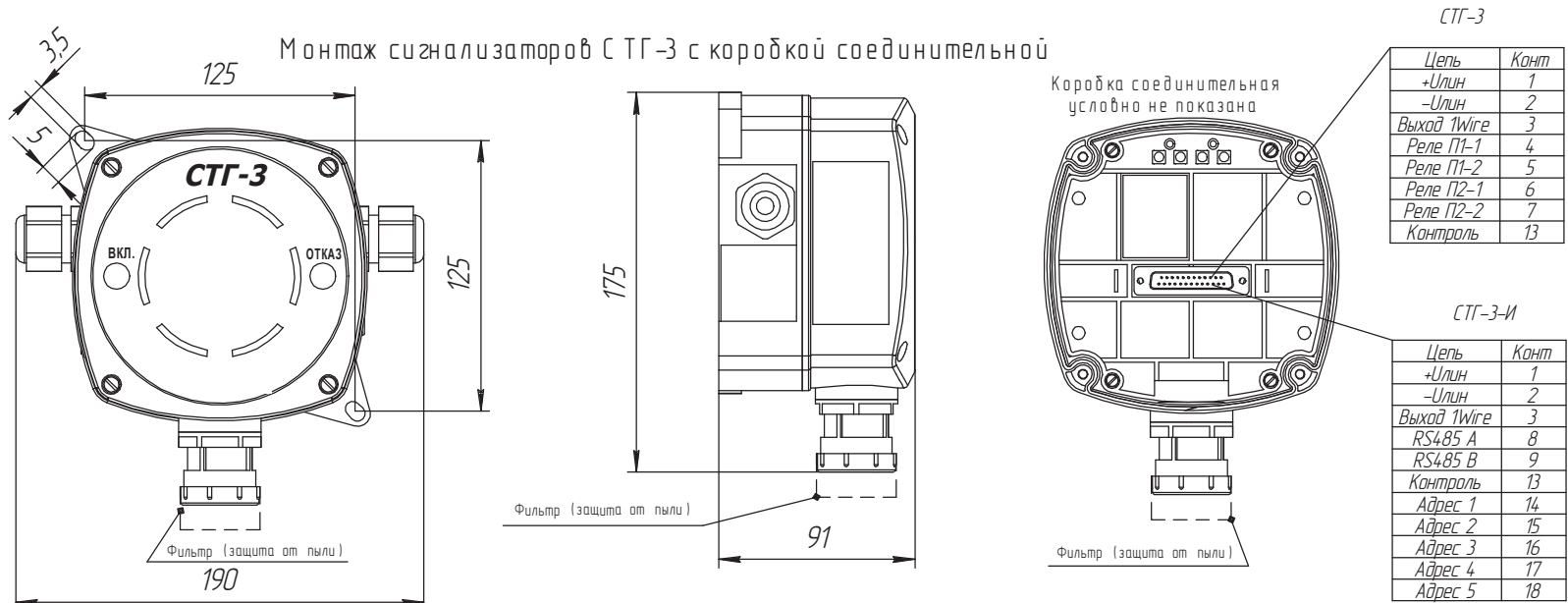
а) сигнализаторы СТГ-3 с ЭХЯ;
