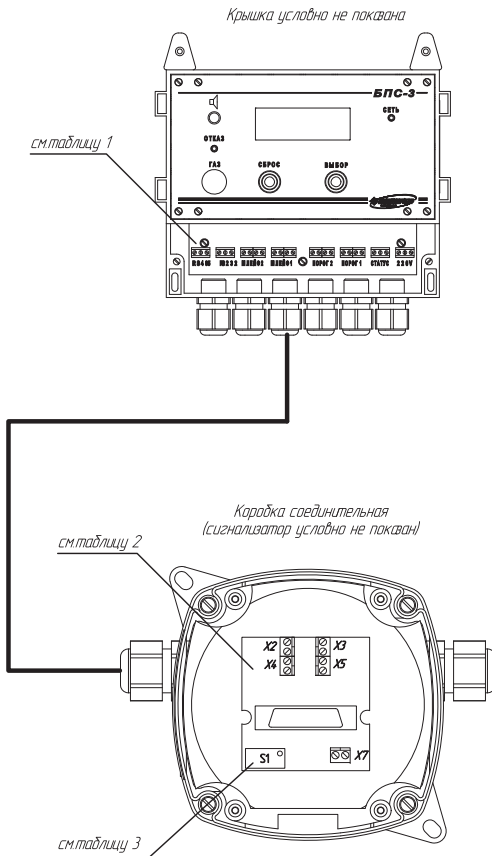
а) сигнализатор СТГ-3-И с блоком БПС-3-И
